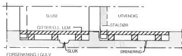
KOTEFORSKJELL MELLOM TILFLUKTS- ROM OG ROM UTENFOR
